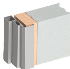
Karmtyp B, foderbildande utsida
