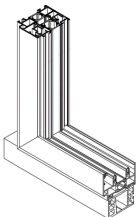
Figur 1 – placering på Schüco basprofil
