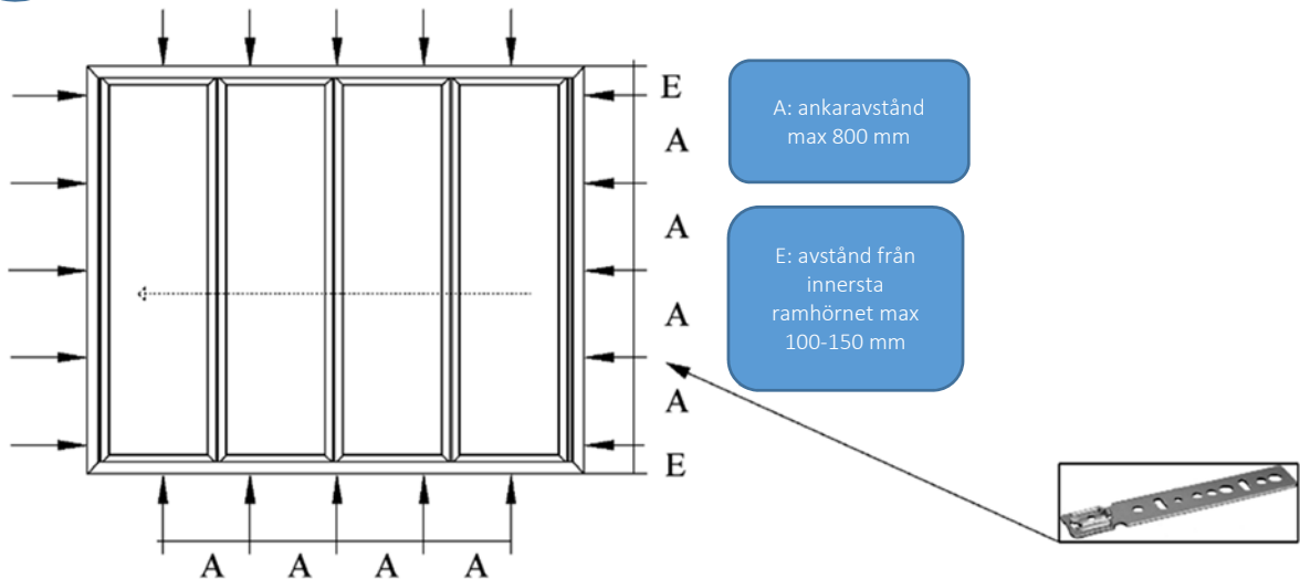
Figur 5–Schüco vridankare
